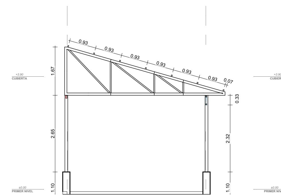
SECCION B-B 1:75
