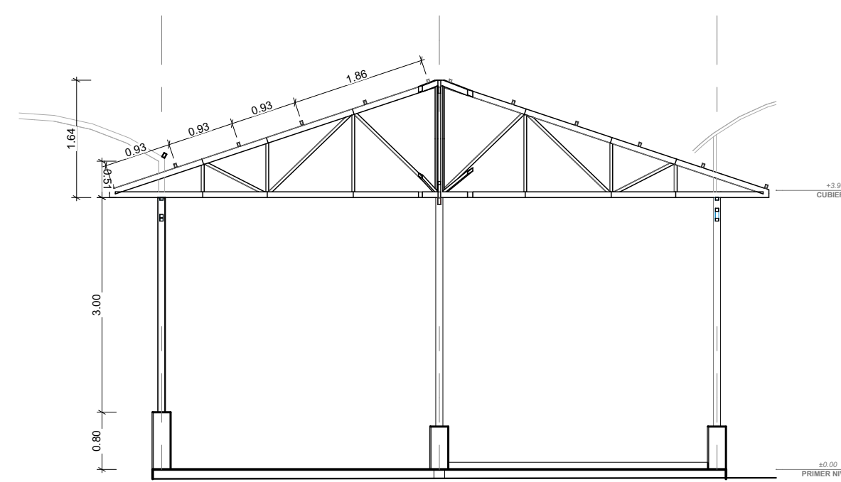
SECCION E-E 1:75
