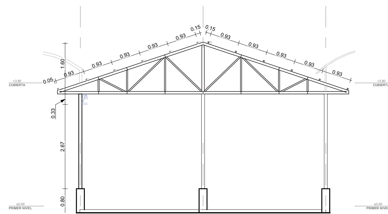
SECCION A-A 1:75
