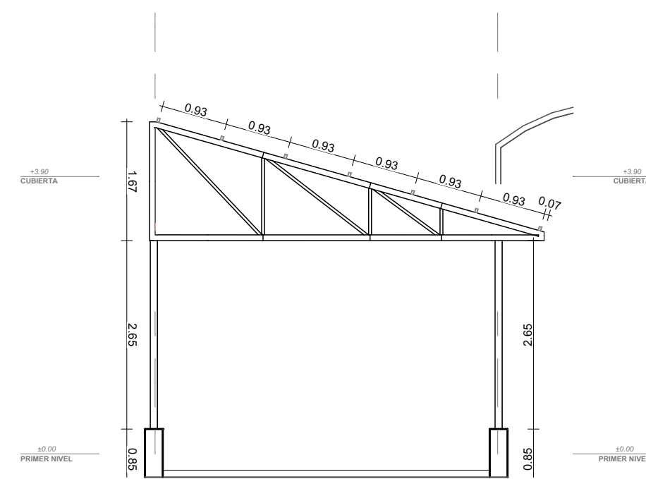
SECCION D-D 1:75
