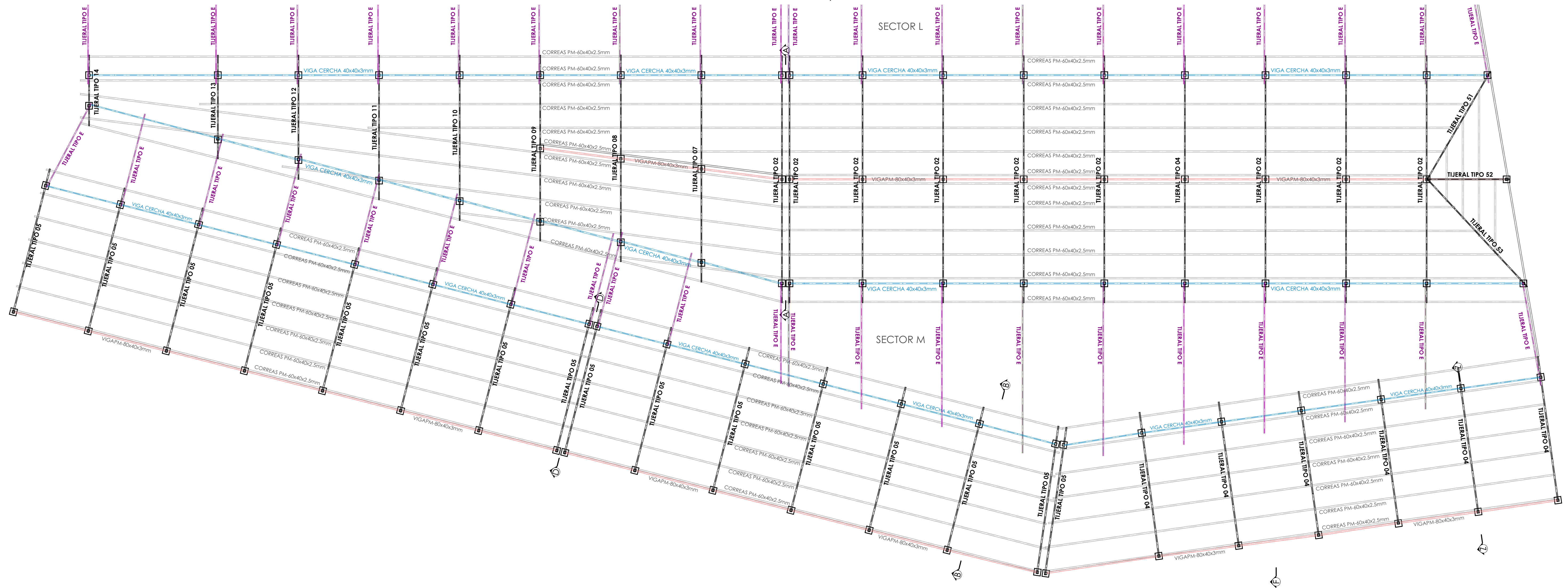
ESTR. CUBIERTA 1:75
